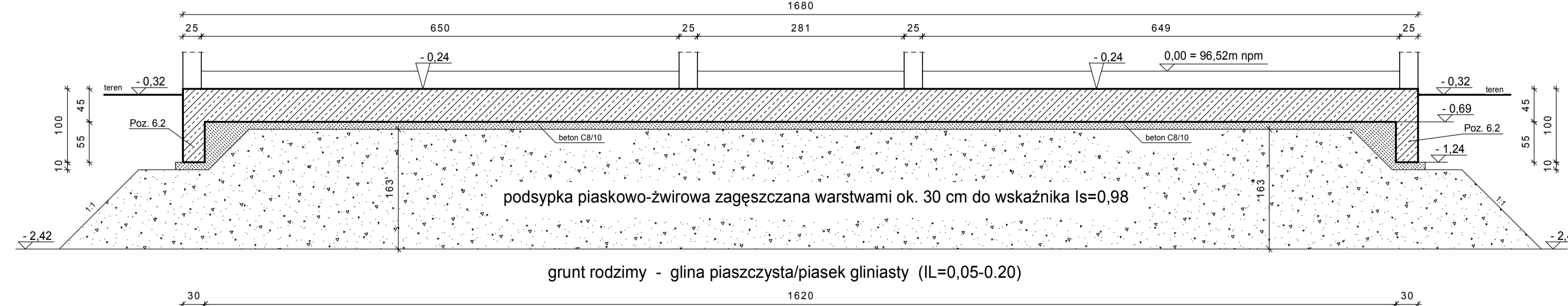
PRZEKRÓJ A-A
