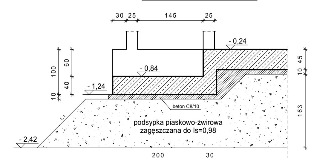
PRZEKRÓJ B-B
