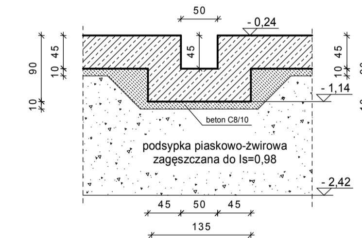
PRZEKRÓJ C-C
